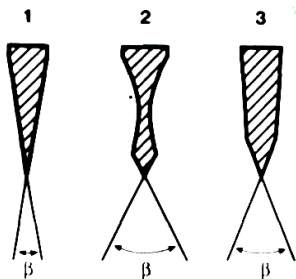
Рис. 8. Основні перетини клинків: 1 – клин; 2 – клин з підводкою; 3 – подвосний клин.
