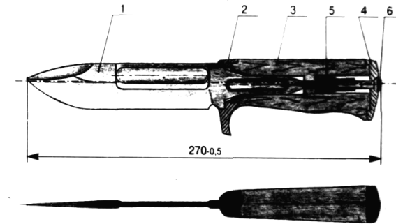
Рис. 6. Будова бойового ножа для метання: 1 – клинок; 2 – обмежувач (перехрестя); 3 – руків'я; 4 – п'ятка; 5 – гайка хвостовика; 6 – гвинт п'ятки.
