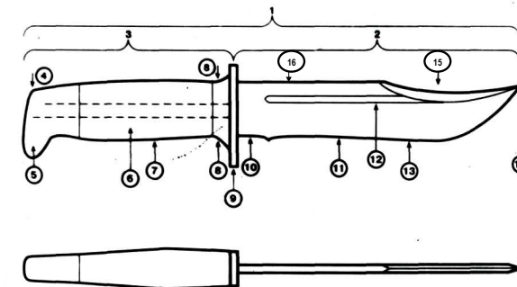
Рис. 7. Складові елементи ножа: 1 – загальна довжина ножа; 2 – довжина клинка; 3 – довжина хвостовика; 4 – п'ятка; 5 – наконечник; 6 – руків'я; 7 – черевце руків'я; 8 – бойові упори; 9 – обмежувач; 10 – основа клинка; 11 – лезо; 12 – ребро жорсткості (жолоб); 13 – ріжуча кромка скосу; 14 – вістря клинка; 15 – скіс обуха; 16 – обух. Зверху - вид з боку, знизу – зверху.
