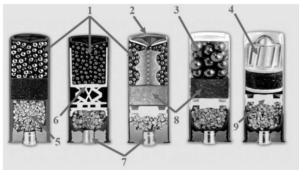
Рис. Мисливські патрони 12 калібру у поздовжньому розрізі: 1 – шріт різних номерів; 2 – гільза; 3 – картеч; 4 – куля; 5 – пороховий заряд; 6 – полімерний клейтух-контейнер; 7 – капсуль; 8 – повстяні клейтухи; 9 – прокладка на пороховий заряд
