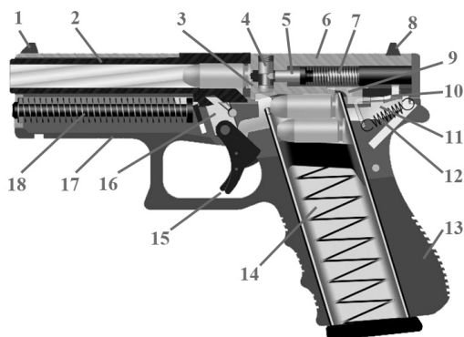
Рис. Схематичне зображення пістолету Глок-23: 1 – мушка; 2 – ствол; 3 – викидач; 4 – автоматичний запобіжник; 5 – ударник з бойком; 6 – кожух-затвор; 7 – пружина ударника; 8 – цілик; 9 – відбивач; 10 – шептало; 11 – спускова тяга; 12 – спускова пружина; 13 – руків'я; 14 – магазин; 15 – спусковий та запобіжний гачки; 16 – замикаючий виступ; 17 – рамка, виконана з ударостійкого пластику; 18 – направляюча вісь зі зворотною пружиною.
