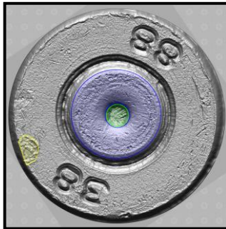
Ілюстрація № 3. Зображення слідів на гільзі, стріляної з пістолета ПБ.
