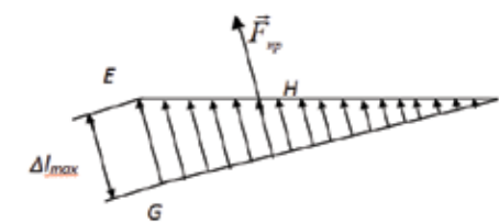
Рис. 2. Схема розподілу інтенсивності пружних сил та їх рівнодійної
