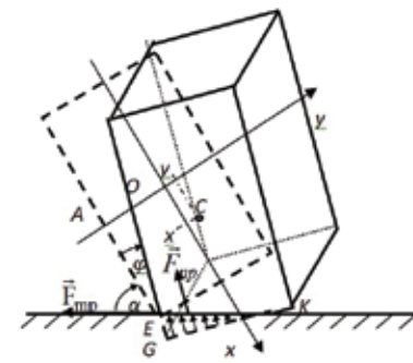
Рис. 1. Схематичне зображення взаємодії елемента ураження з металевою пластинною на етапі проникнення
