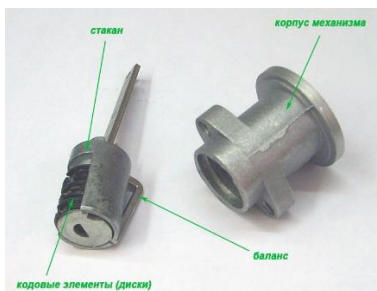
Рисунок 10. Основні механізми дискового замка.
